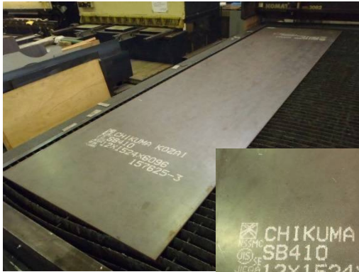
胴板・鏡板 SB410 t=12
