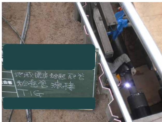
現場溶接中
