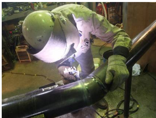
工場内プレハブ加工中
