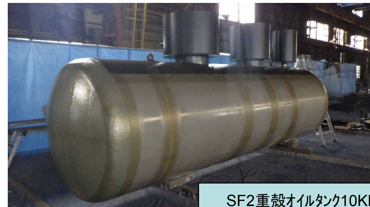
小型圧力容器 設計・製作 させて頂きました
