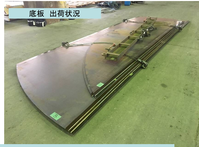
80㎡消火水タンク(工場半加工) φ6,790*4,200H
