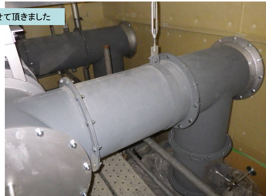
油用クーラーコイル 2つ 製作させて頂きました SUS304L-TPS sch80
