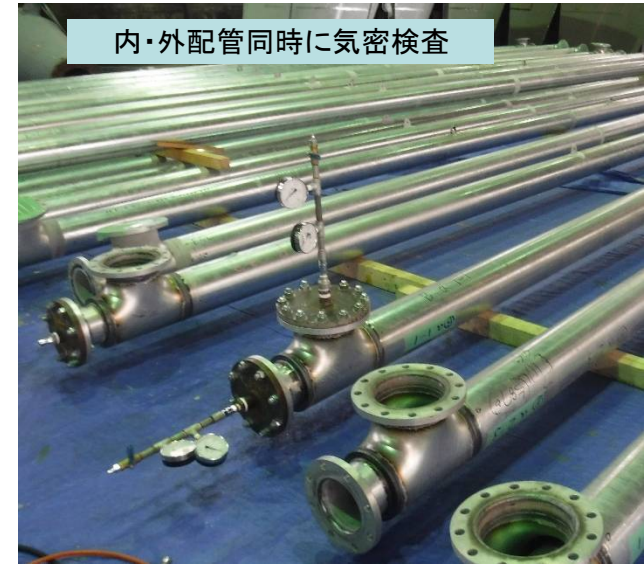
外部配管φ200
