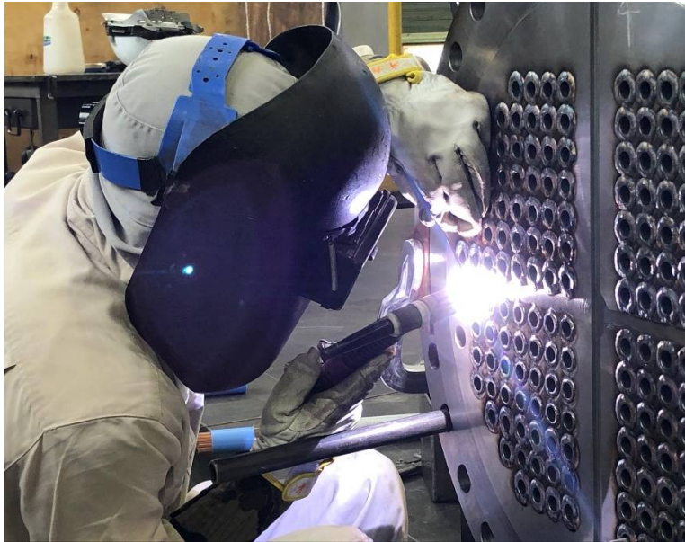
温水発生器 第1種圧力容器 設計製作させて頂きました 胴 SB410 伝熱管 STB-340S 最高使用圧力 1次側 4.0Mpa
