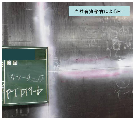
現場溶接部・接合部の取り合い確認
