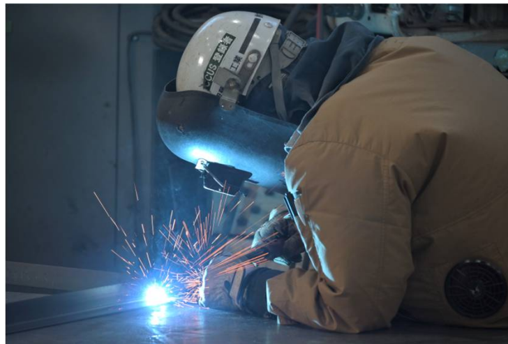
SUS304製 水素バッファータンク(9m 3 )2基 第2種圧力容器 Φ1,700×L3,400 (サドル部素材はSS) 設計製作させて頂きました
