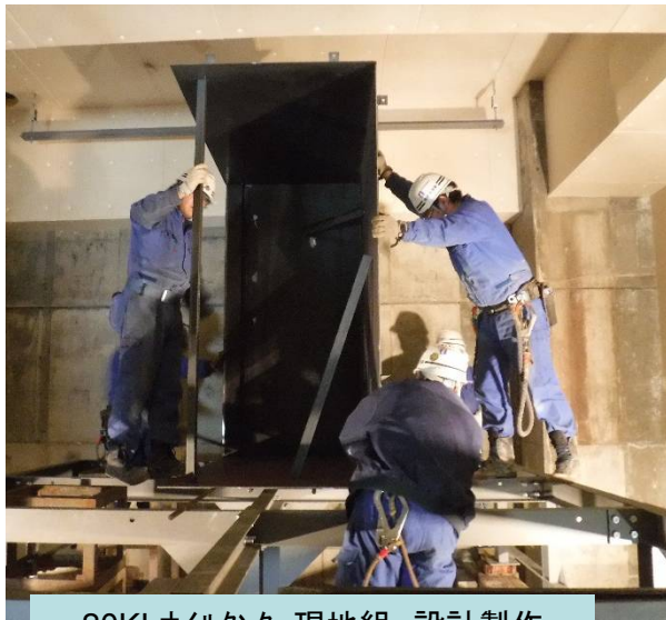
20KLオイルタンク 現地組 設計製作 据付、組立溶接をさせて頂きました
